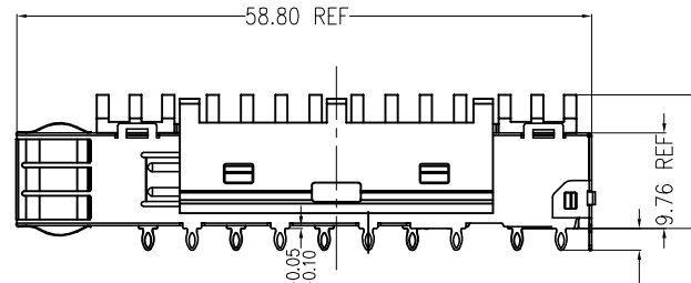
正视图
