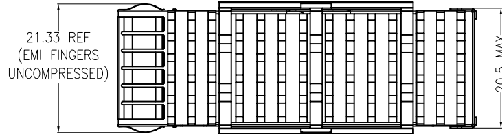
俯视图
