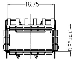
侧视图
